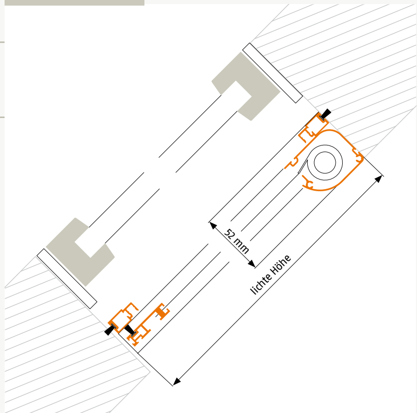
Vertikalschnitt
