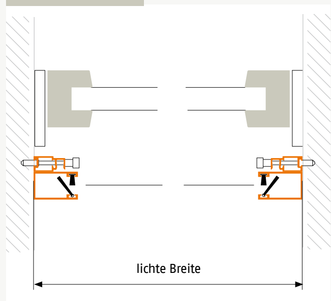
Horizontalschnitt
